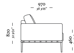
1 Lugar com 1 Braço D/E 1070 x 970 x 820mm
