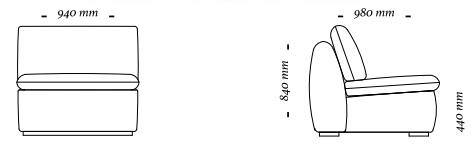
Poltrona 900mm s/ br 940x980x840mm
