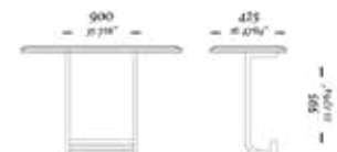
Mesa de apoio Tampo laminado chanfrado 900 x 425 x 395mm
