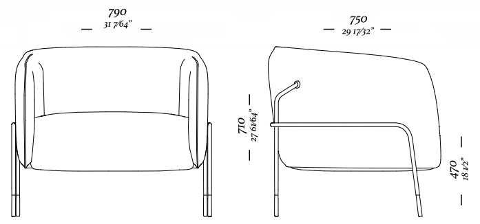
Poltrona 790x750x 710 mm
