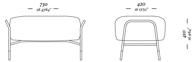
Banqueta 730x420x410 mm
