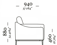
Sofá 4 lugares C/ 2BR 2900x940x880mm
