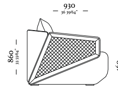
Mod c/ oi br D/E Assento 900mm 970 x 930 x 860mm
