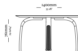
Mesa com diametro de 1400 mm
