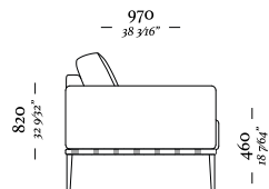
3 Lugares com 2 Braços 2110 x 970 x 820mm
