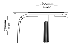
Mesa com diametro de 1600 mm e giratorio
