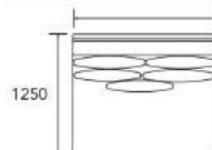
MÓDULO S/ BRAÇO 850 / 900 / 1000 / 1100 / 1200 / 1300
