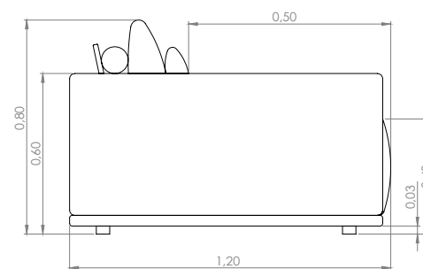
Módulo fechado
